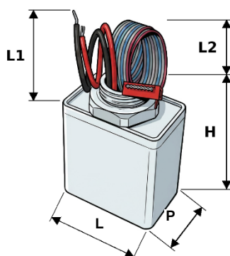
ALLT.M.D.12-24V DC
